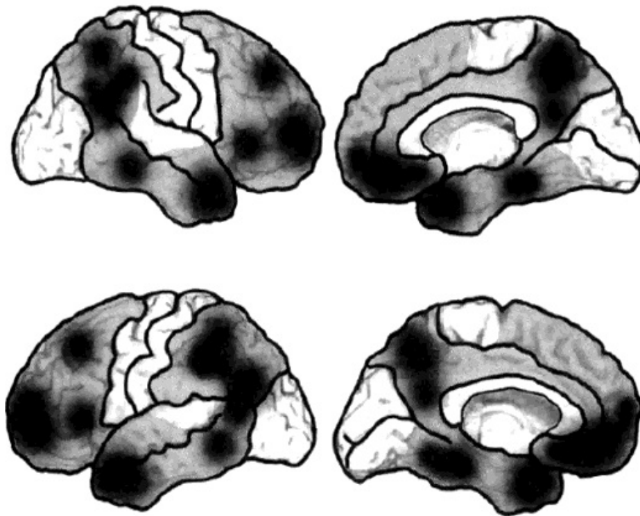
Figura 9.2. La tarea de coordinar las diversas imágenes que genera el proceso de percepción y recuerdo en curso cuenta con la ayuda de las RCD situadas en el interior de las cortezas de asociación que no están sombreadas. La localización aproximada de las principales RCD viene sugerida en los esquemas: las cortezas polar y medial del lóbulo temporal, las cortezas mediales prefrontales, las confluencias temporoparietales y las cortezas posteromediales (CPM). Hay otras regiones de este tipo sin lugar a dudas. La mayoría de las RCD representadas en esta figura forman parte también de la «red neural por defecto» de Raichle, que trataremos más adelante en este capítulo.
