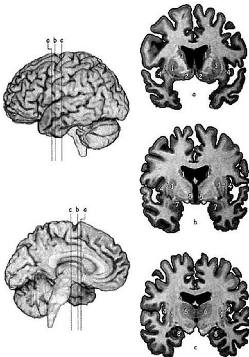
Figura A. 2. Los diagramas de la izquierda representan las reconstrucciones en tres dimensiones del encéfalo humano visto desde las perspectivas lateral (externa) y medial (interna). Los diagramas de la derecha muestran las tres secciones del volumen encefálico. Las secciones se obtienen siguiendo las líneas que aparecen marcadas en la ilustración con las letras a, b y c. Las secciones revelan un número importante de estructuras situadas por debajo de la superficie: (1) los ganglios basales; (2) el cerebro anterior basal; (3) el claustró; (4) la corteza insular; (5) el hipotálamo; (6) el tálamo; (7) la amígdala; (8) el hipocampo. La corteza cerebral cubre la superficie completa de los dos hemisferios cerebrales, incluyendo cada circunvolución hasta el fondo. En las secciones, la corteza cerebral aparece como un reborde oscuro que se distingue fácilmente de la sustancia blanca que tiene debajo. Las áreas en negro situadas en el centro de las secciones corresponden a los ventrículos laterales.
