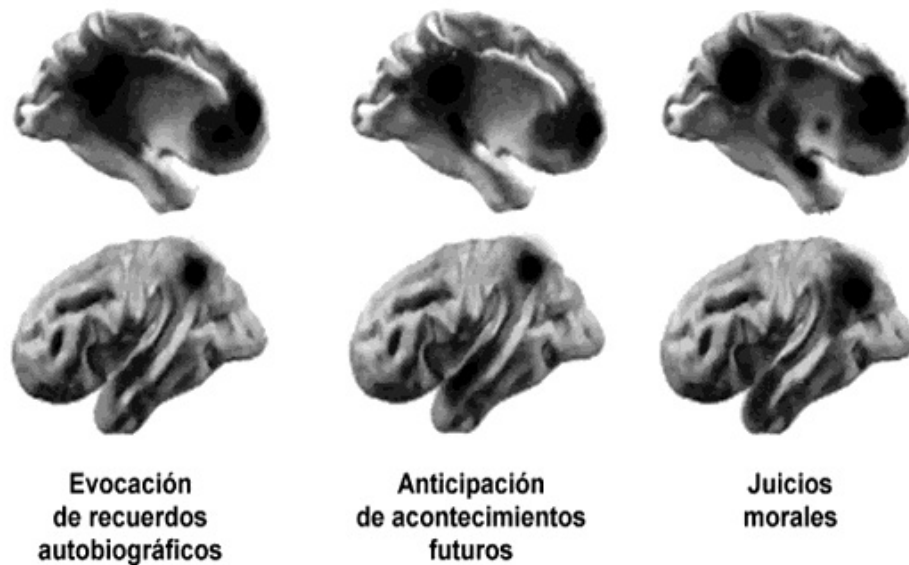
Figura 9.5. La corteza posteromedial (CPM), junto con otras regiones de convergencia y divergencia, se hallan prominentemente activadas al realizar una variedad de tareas autorreferenciales tal como lo muestran estas imágenes obtenidas con la técnica de imagenía funcional. De este tipo de tareas forman parte la evocación de recuerdos autobiográficos, la anticipación de acontecimientos futuros y la formación de juicios morales.
