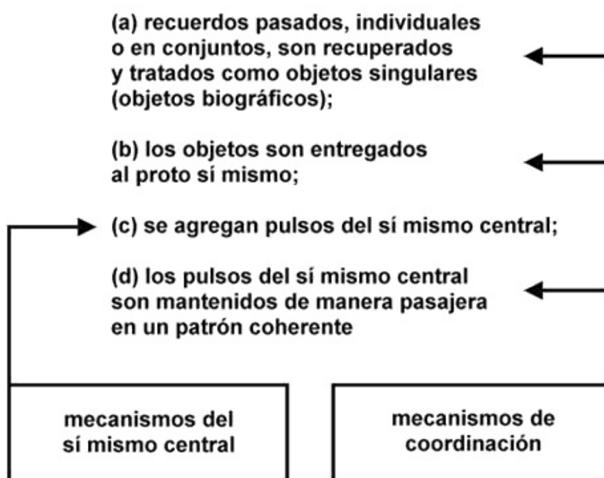
Figura 9.1. Mecanismos neurales del sí mismo autobiográfico.
