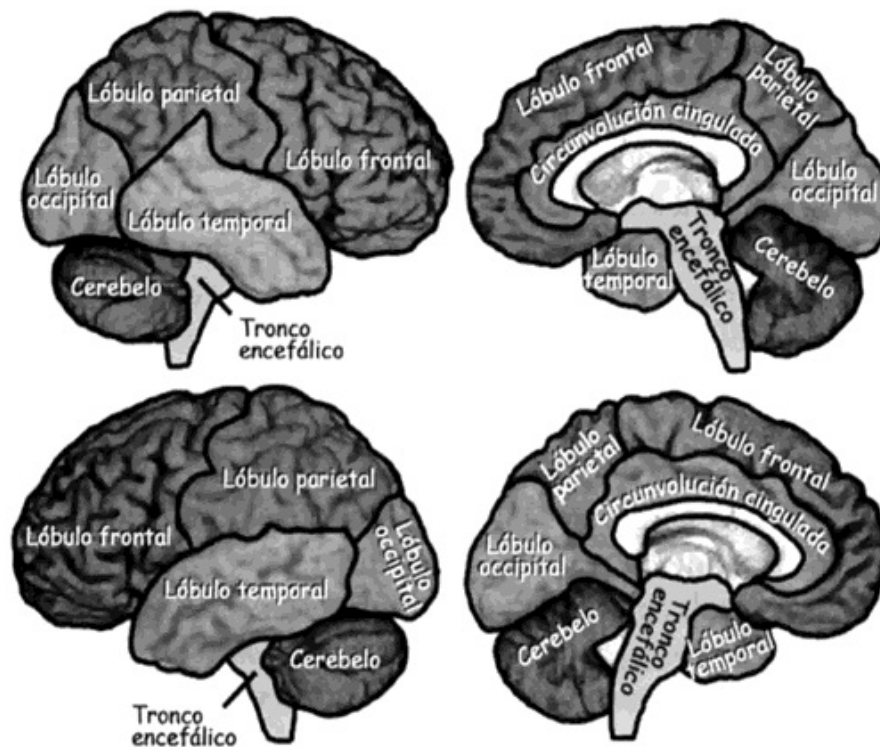
Figura A. 1. Las reconstrucciones en imágenes tridimensionales de los datos obtenidos a través de la técnica de resonancia magnética muestran la arquitectura a gran escala del cerebro humano. Las secciones laterales (vistas externas) de ambos hemisferios, derecho e izquierdo, aparecen en esta ilustración en los diagramas de la izquierda, en tanto que las secciones mediales (vistas internas) aparecen en los diagramas de la derecha. La estructura blanca curvada que aparece en los diagramas de la derecha corresponde al cuerpo calloso.
