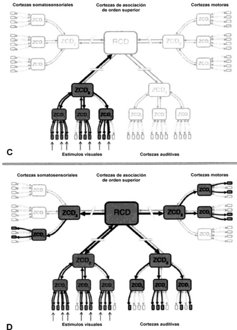
Figura 6.2. Utilización de la arquitectura de convergencia y divergencia para reconocer recuerdos suscitados por un estímulo visual específico. En los esquemas A y B, un cierto estímulo visual entrante (un conjunto selectivo de pequeños rectángulos sombreados) incita a la actividad en las zonas de convergencia y divergencia ZCD1 y ZCD2 (flechas y rectángulos sombreados). En el esquema C, la actividad entrante activa regiones de convergencia y divergencia específicas, y en el esquema D, la retroacción genera exposiciones en el «espacio de imagen» así como movimiento (conjunto selectivo de pequeños rectángulos sombreados).
