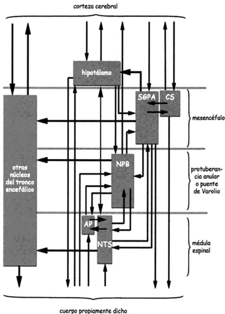
Figura 8.3. Los núcleos del tronco encefálico que intervienen en la generación del sí mismo central.
