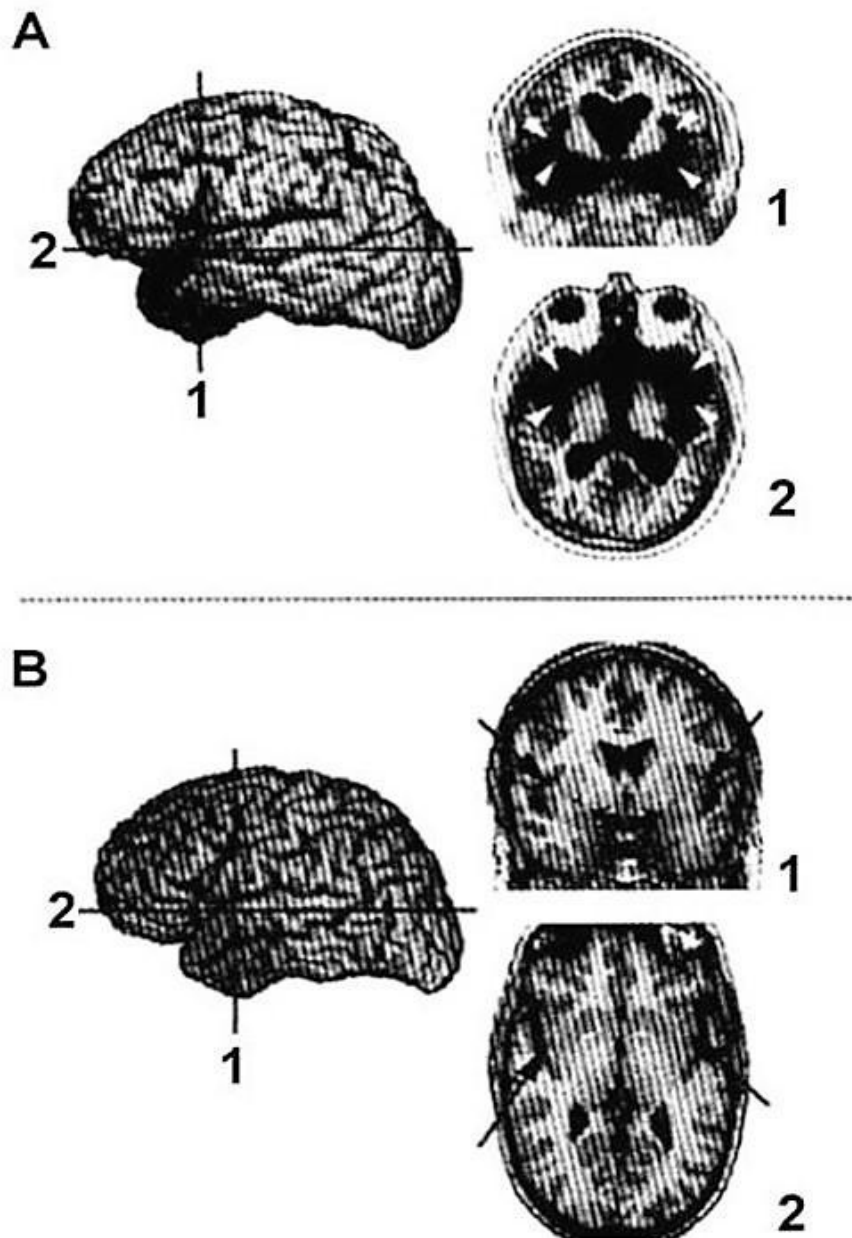
Figura 3.2. La parte de arriba (A) muestra un escáner obtenido por medio de resonancia magnética de un paciente afectado por una lesión completa de las cortezas insulares (ínsula), tanto en el hemisferio izquierdo como en el derecho. En la parte de la izquierda se muestra una reconstrucción del cerebro del paciente. En la parte de la derecha, se muestran dos cortes del cerebro (marcados con los números 1 y 2) tomados siguiendo los ejes horizontal y vertical indicados sobre la reconstrucción del cerebro en la parte izquierda e indicados con los números 1 y 2 respectivamente. El área que aparece en negro corresponde al tejido cerebral destruido por la enfermedad. Las flechas blancas señalan las localizaciones en las que deberían de haber aparecido las ínsulas. En la parte B, situada abajo en la figura se muestra un cerebro normal en tres dimensiones y dos cortes tomados siguiendo los mismos ejes que en el caso anterior. Las flechas negras señalan, en este caso, la ubicación de las cortezas insulares normales.
