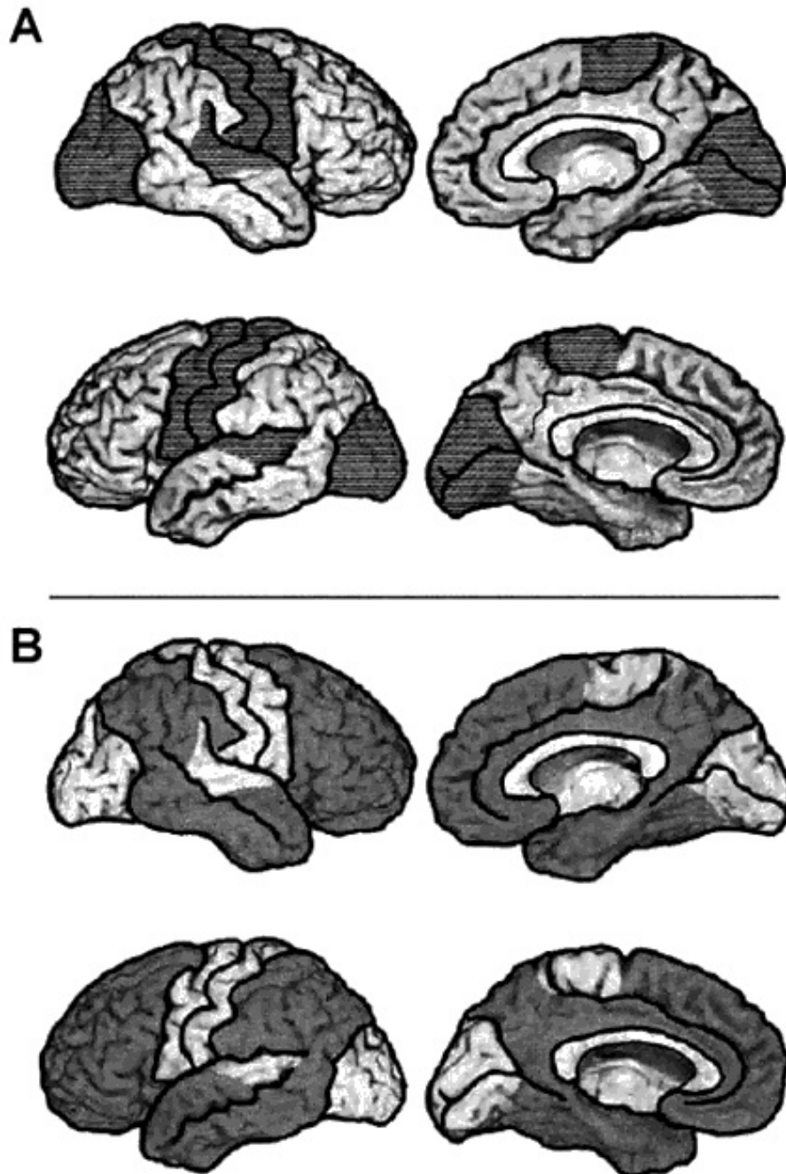
Figura 6.3. El espacio de imagen (marcado) y el espacio de las disposiciones (no marcado) en la corteza cerebral. Este espacio de las imágenes aparece representado en las áreas sombreadas de los cuatro dibujos de A en la parte superior de la figura, junto con la corteza motora primaria. El espacio de las disposiciones se representa en los cuatro dibujos de B, en la parte inferior de la Figura, y aparece también sombreado.
