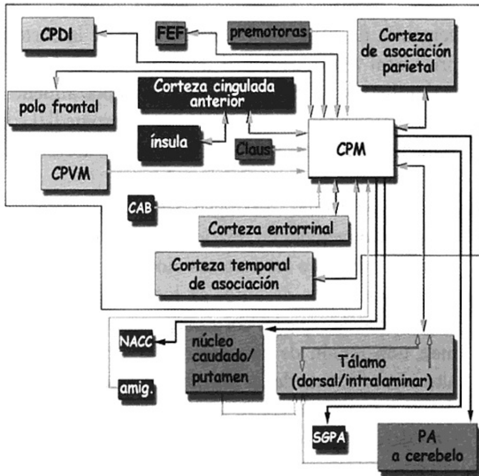
Figura 9.4. La configuración de las conexiones neuronales de entrada y salida de las cortezas posteromediales, tal como se determinó en un estudio realizado con monos. (CPDI: Corteza prefrontal dorsolateral); FEF: campos oculares frontales; CPM: corteza posteromedial; CPVM: corteza prefrontal ventromedial; CAB: Cerebro anterior basal; Claus: claustrum; NACC: núcleo accumbens; amig.: amígdala; SGPA: sustancia gris periacueductal; PA: protuberancia anular (puente de Valerio).
