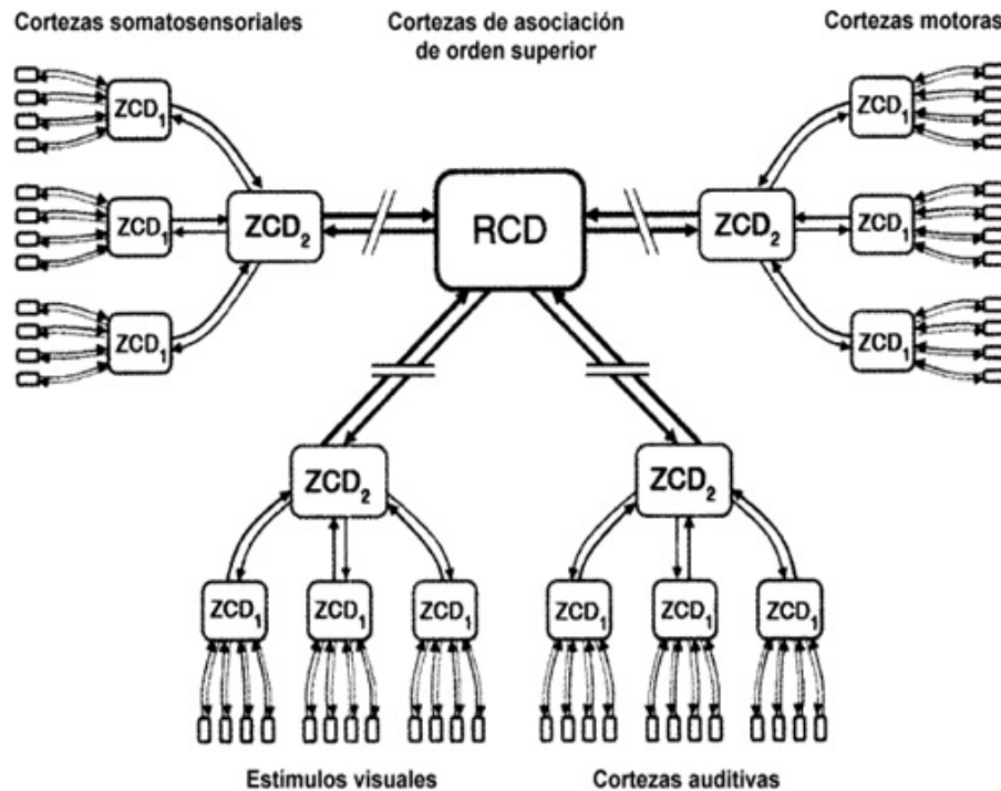
Figura 6.1. Esquema de la arquitectura de convergencia y divergencia, en el que se indican cuatro niveles jerárquicos. El nivel cortical primario está indicado por medio de rectángulos pequeños, y tres niveles de convergencia-divergencia (rectángulos mayores) se indican con las letras ZCD1, ZCD2 y RCD. Entre los niveles ZCD (zonas de convergencia-divergencia) y RCD (regiones de convergencia-divergencia), indicadas con flechas discontinuas, son posibles numerosas zonas de convergencia y divergencia (ZCD) intermedias. Obsérvese que a lo largo de toda la red, a cada proyección hacia delante le corresponde una proyección de retorno (flechas).
